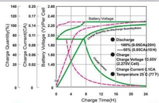
نمودار منحنی شارژ در حالت آماده بکار
