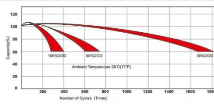
نمودار چرخه عمر نسبت به عمق دشارژ
