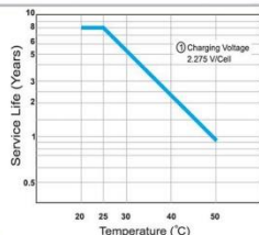
نمودار طول عمر در دمای متغیر
