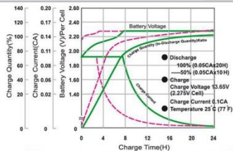
نمودار منحنی شارژ در حالت آماده بکار
