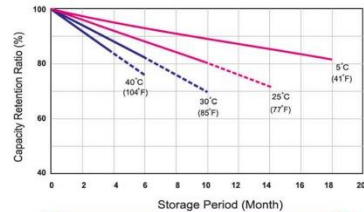
نمودار مشخصه حفظ ظرفیت
