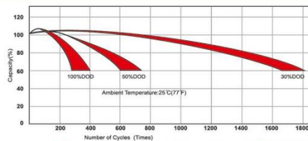
نمودار چرخه عمر نسبت به عمق دشارژ
