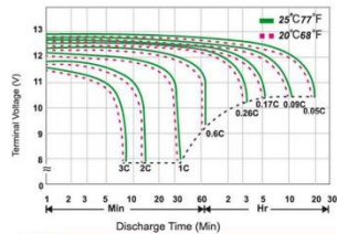
نمودار دشارژ
