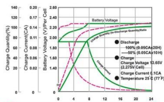
نمودار منحنی شارژ در حالت آماده به کار
