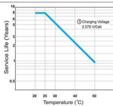
نمودار طول عمر در دمای متغیر
