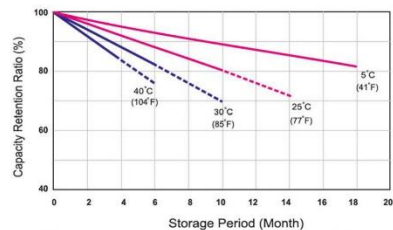
نمودار مشخصه حفظ ظرفیت
