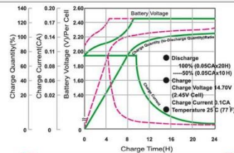
نمودار منحنی شارژ در حالت استفاده
